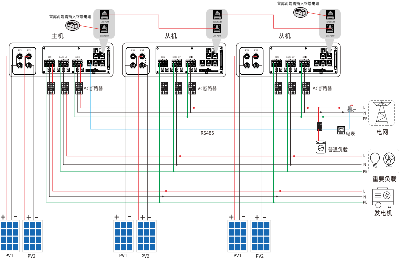
单相并机接线图
